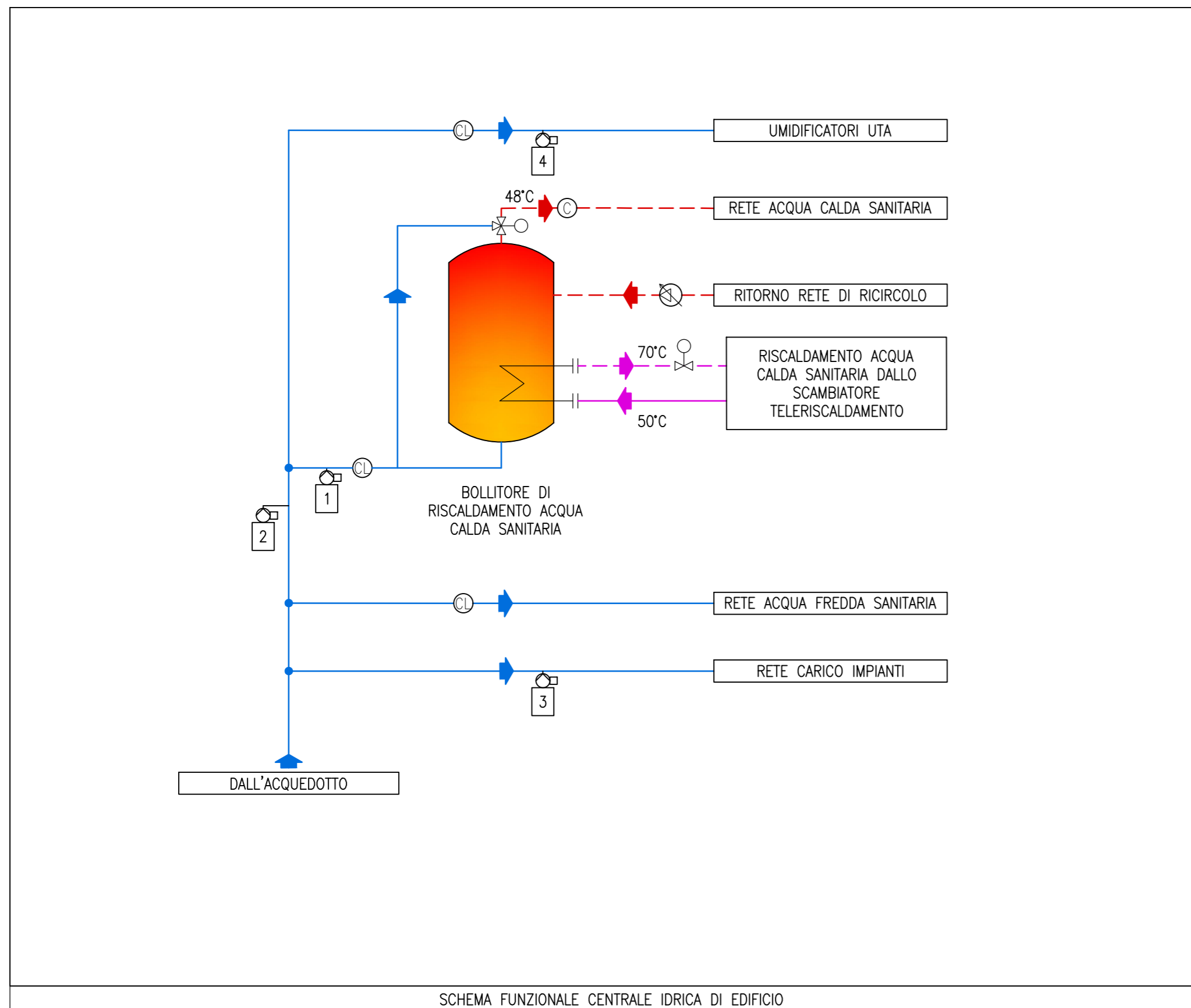
SCHEMA FUNZIONALE CENTRALE IDRICA DI EDIFICIO
